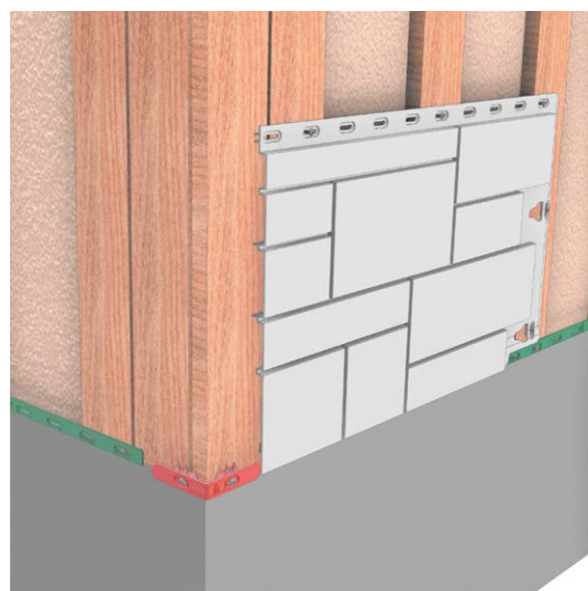
Рис. 20 Монтаж первой панели
