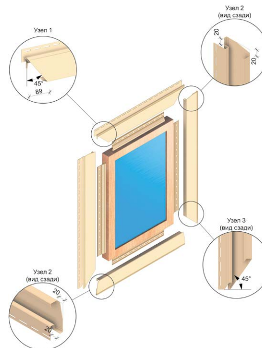
Рис. 11 Обрамление оконного проёма при помощи наличника 89 мм.
