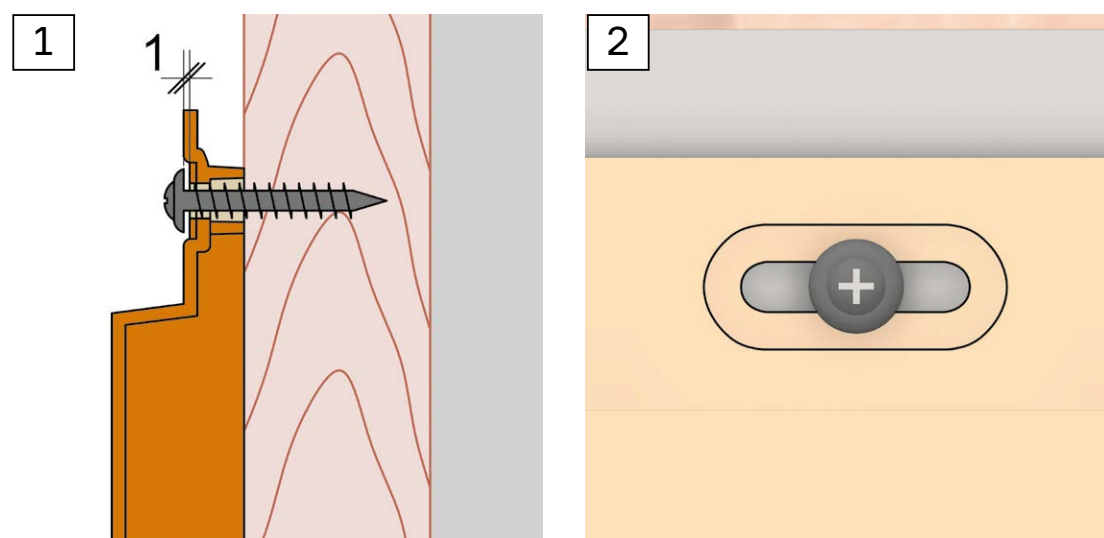
Рис. 2 Схема фиксации фасадных и цокольных панелей Döcke
