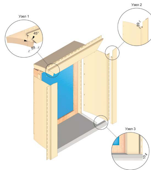
Рис. 16 Обрамление оконного проёма при помощи наличника 89 мм с откосом 254 мм.
