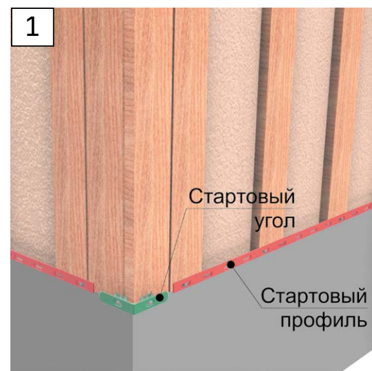
Рис. 9 Установка стартовых профилей и стартовых углов
