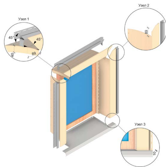
Рис. 15 Обрамление оконного проёма при универсального околооконного профиля с соответствующим J-профилем (таблица 4) при наличии металлического отлива.
