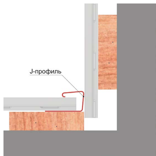
Рис. 19 Монтаж обрешётки под внутренний угол
