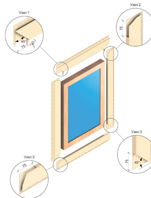
Рис. 12 Обрамление оконного проёма при помощи наличника 75 мм.
