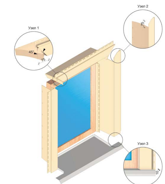
Рис. 18 Обрамление оконного проёма при помощи околооконного профиля 75/200/13 мм (только для ЭДЕЛЬ) при наличии металлического отлива.
