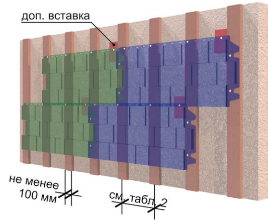
Рис. 5 Вертикальная обрешётка под фасадные панели Döcke FELS, BURG и цокольные панели ЭДЕЛЬ
