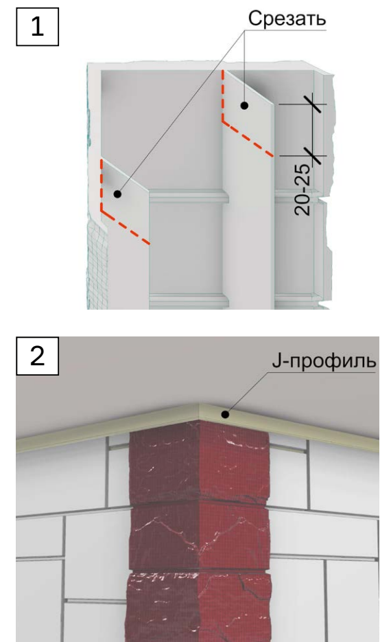
Рис. 26 Примыкание внешнего угла Döcke к карнизному свесу.
