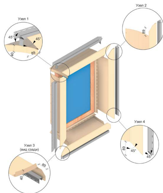
Рис. 14 Обрамление оконного проёма при универсального околооконного профиля с соответствующим J-профилем (таблица 4).
