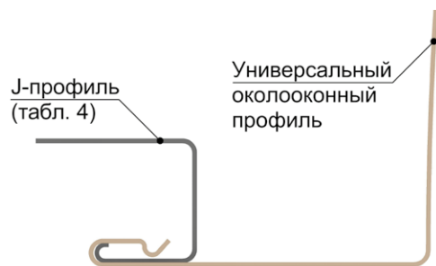
Рис. 13 Соединение универсального околооконного профиля с соответствующим J-профилем (таблица 4).
