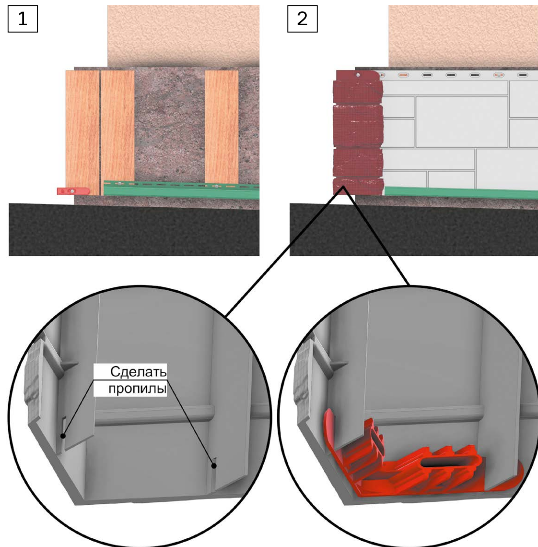
Рис. 23 Отделка цоколя с перепадом высоты
