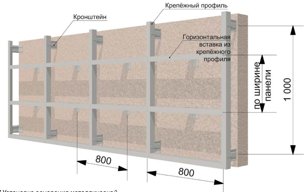
Рис. 7 Установка основания металлической обрешётки под фасадные и цокольные панели Döcke (вертикальные вставки не показаны (см. рис. 8))
