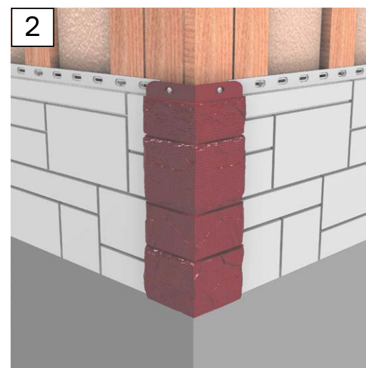
Рис. 21 Монтаж первого ряда панелей
