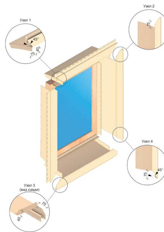
Рис. 17 Обрамление оконного проёма без отлива при помощи околооконного профиля 75/200/13 мм (только для ЭДЕЛЬ).
