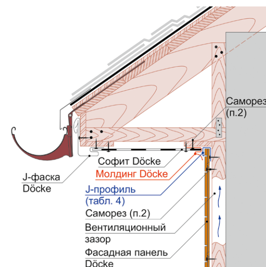
Рис. 24 Примыкание фасадных панелей Döcke к карнизному свесу.
